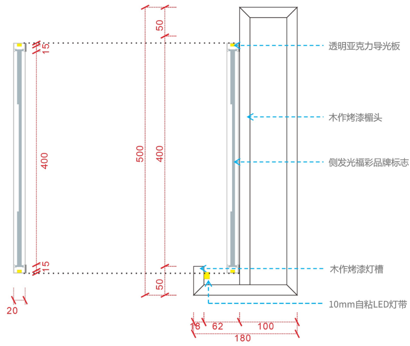
500mm高烤漆板造型门头剖面尺寸图
