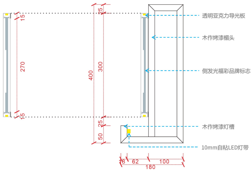
400mm高烤漆板造型门头剖面尺寸图
