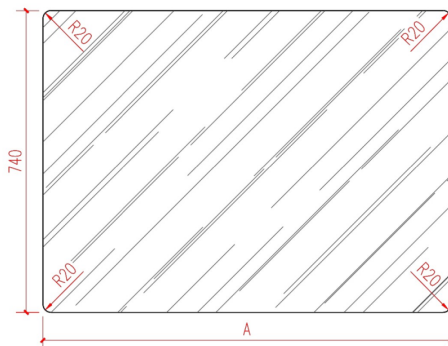
俯视图
