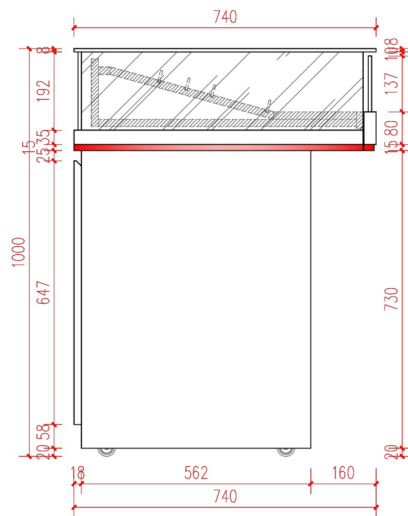
左侧视图
