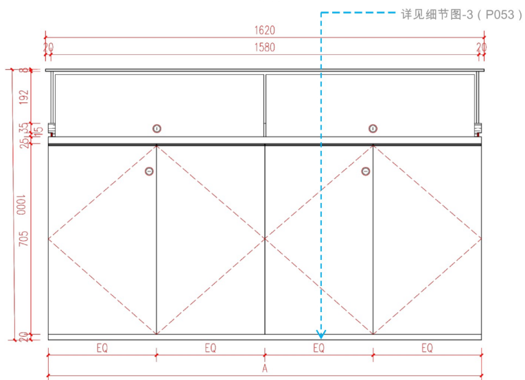
背立面图
