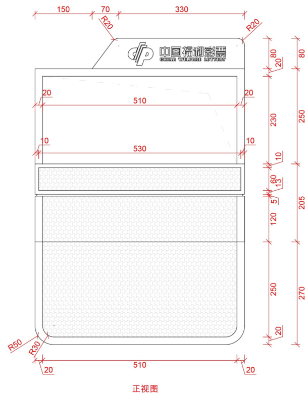
正视图
