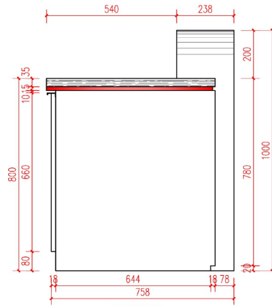
左侧视图
