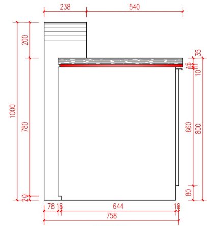
右侧视图
