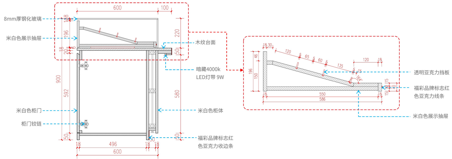
A7带灯箱岛台柜剖面图
