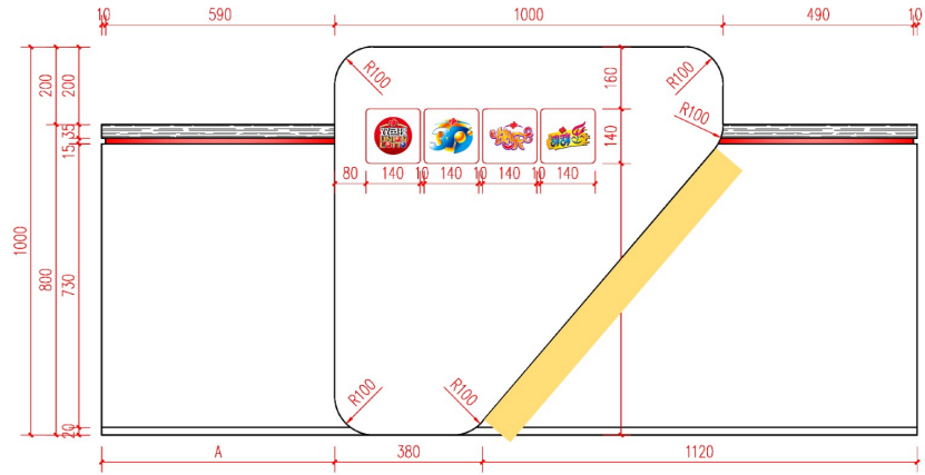
正立面图
