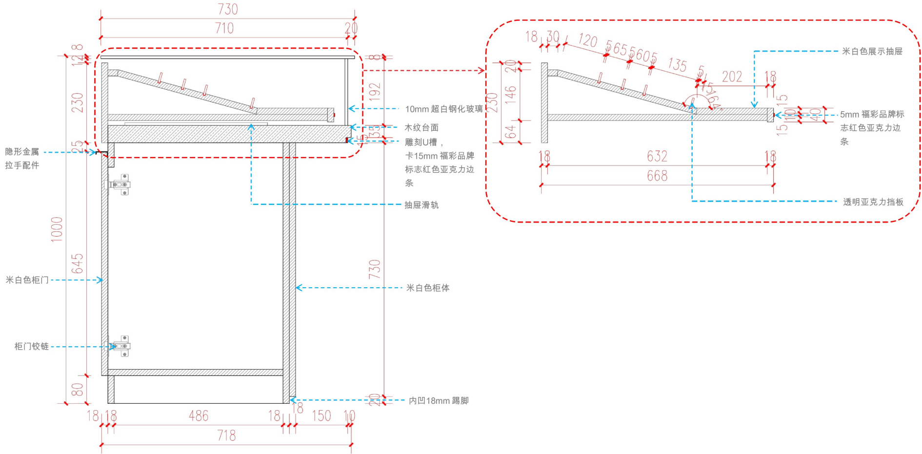
A2即开票抽屉柜剖面图
