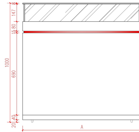
正立面图
