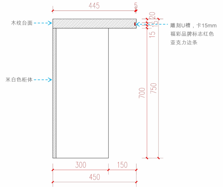
B2配套独立桌剖面图
