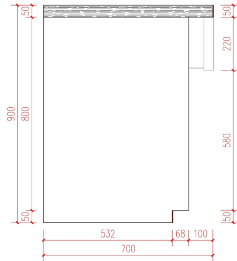
左侧视图
