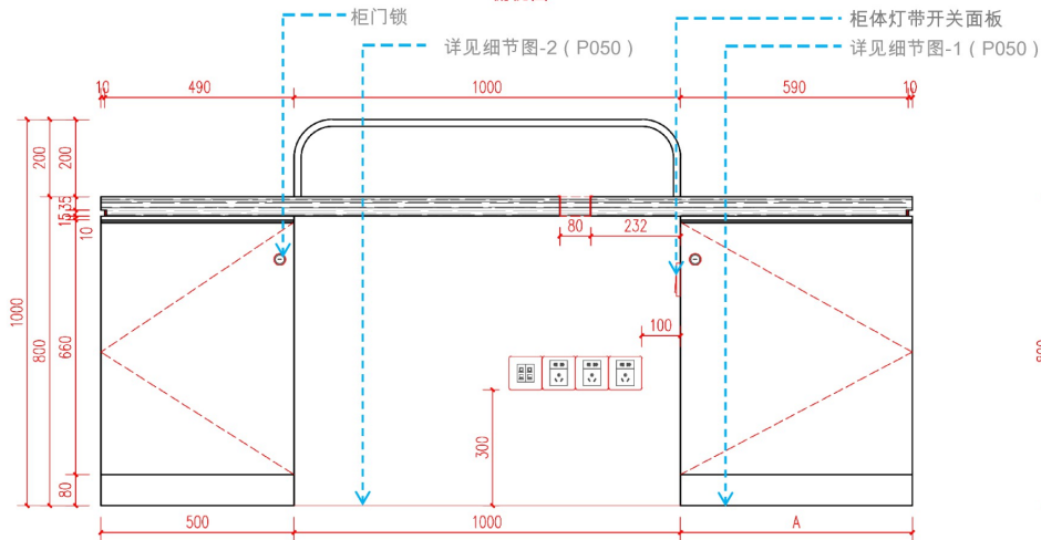
背立面图
