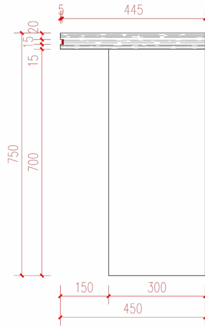
右侧视图
