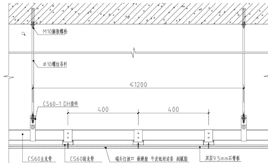
石膏板吊顶工艺示意
