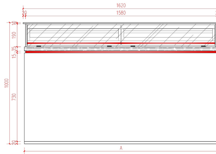
正立面图
