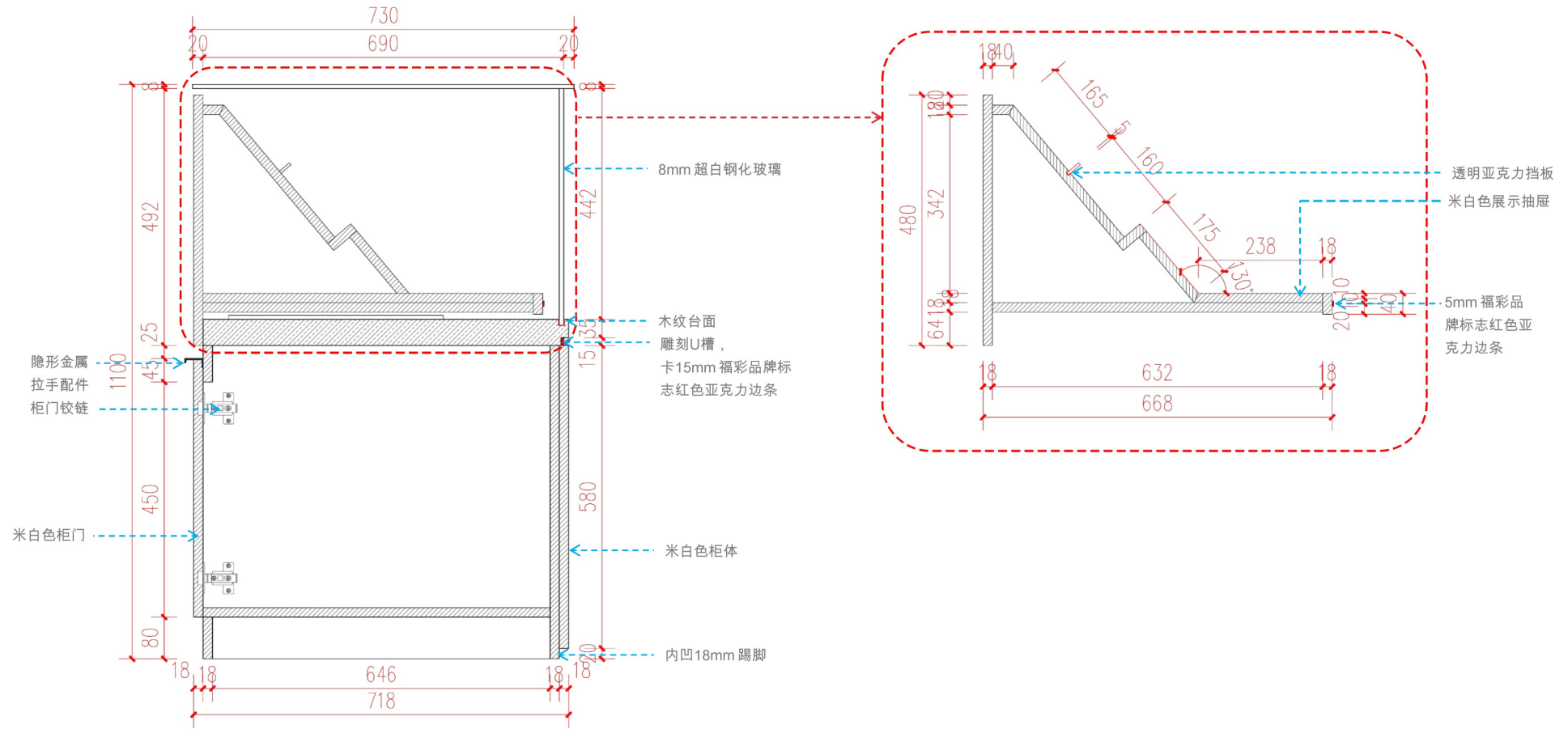
A3即开票玻璃柜剖面图
