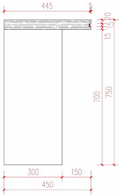
左侧视图
