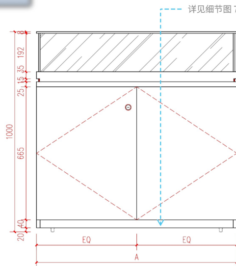
背正立面图
