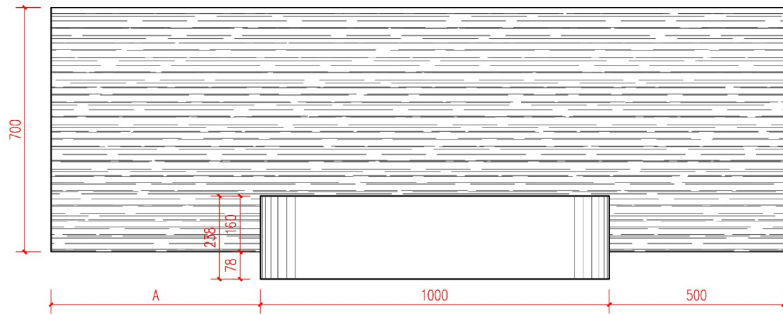
俯视图
