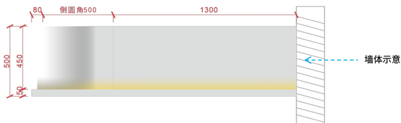
500mm高烤漆板造型门头长度尺寸规范示意图（中岛式放置）
