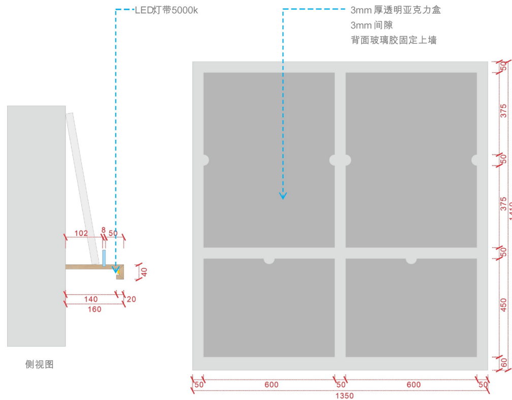
海报活动宣传亚克力展示盒尺寸图
