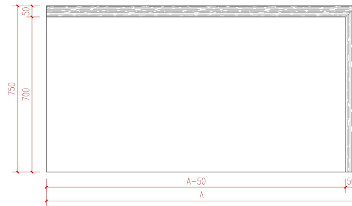
背立面图
