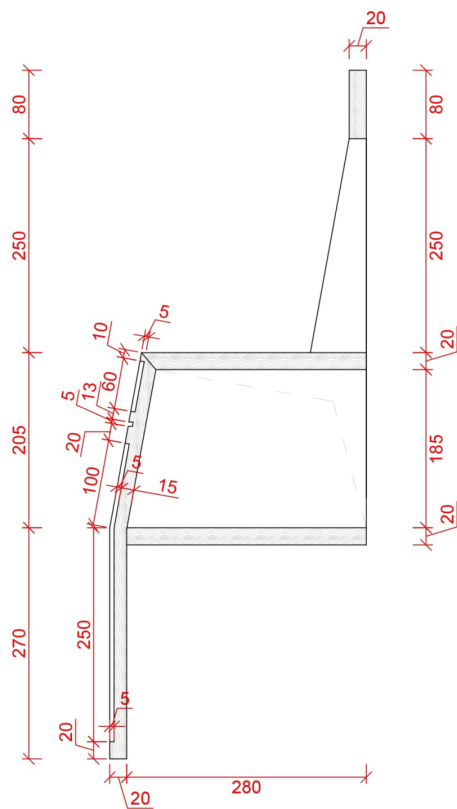
侧视图结构图
