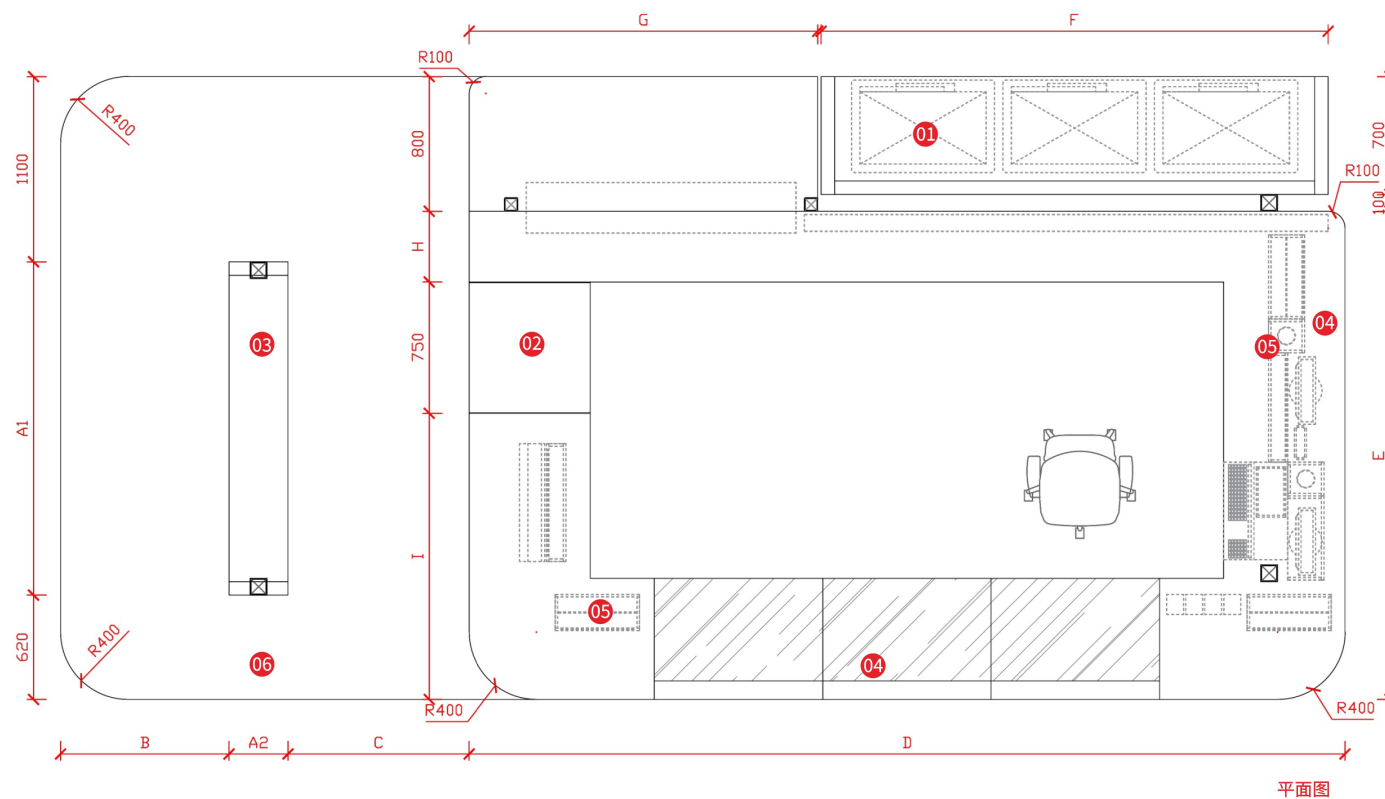
平面图
